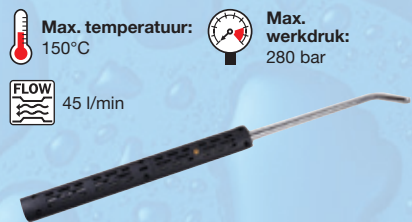
Gebogen lans - open isolatie - 1/4" BSPT inlaat/uitlaat
